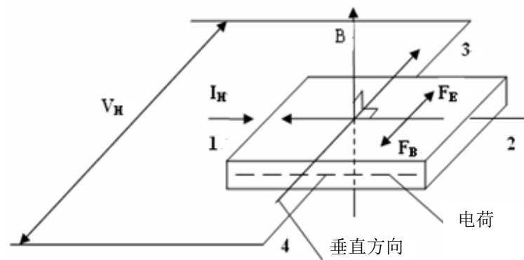
霍尔效应及其电气参数
